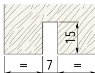
Detail vyfrézovaného dveřního křídla
