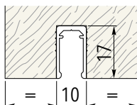
Detail vsunutého ochranného profilu
