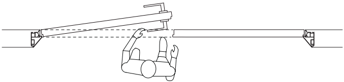
LEVÉ DVEŘE OTEVÍRANÉ DOVNITŘ - PRAVÉ FIXNÍ
