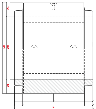
POHLED SESHORA / PODÉLNÝ ŘEZ
