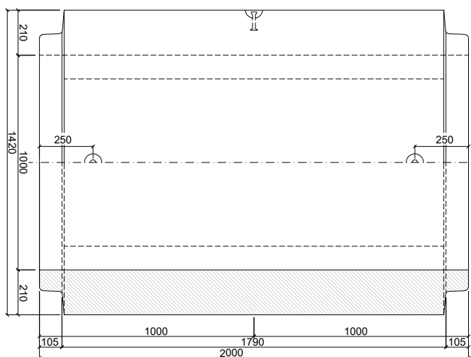
PATKOVÁ TROUBA TZP-ZP 100/200 DD
