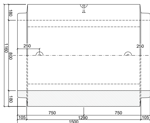
PATKOVÁ TROUBA TYP-ZP 80/150 DD
