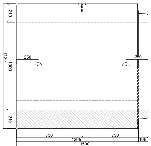
PATKOVÁ TROUBA TZP-SP 100/150 KD
