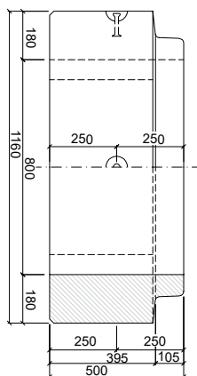
PATKOVÁ TROUBA TZP-ZP 80/50 KD
