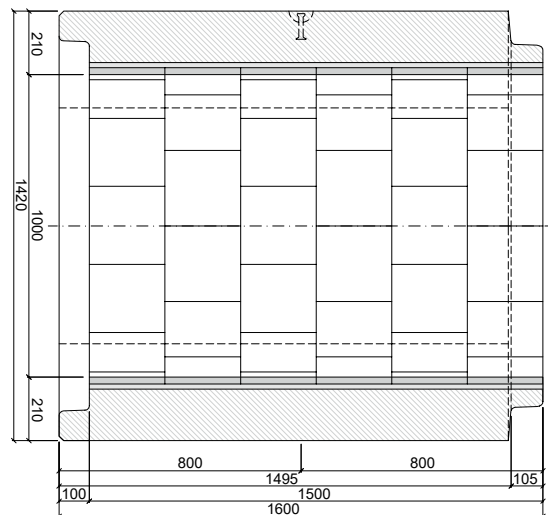
PATKOVÁ TROUBA TZP-SP 100/150 HDOC
