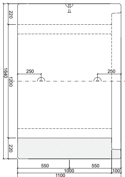
PATKOVÁ TROUBA TZP-SP 120/100 KH
