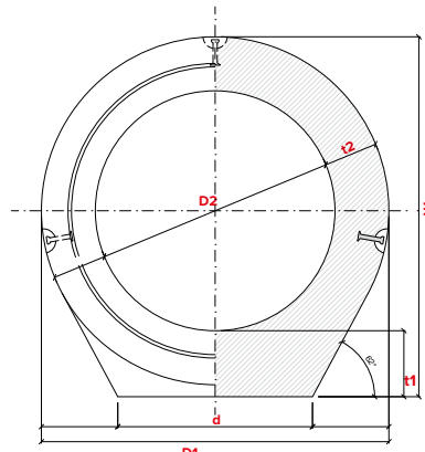
POHLED ČELNÍ / PŘÍČNÝ ŘEZ
