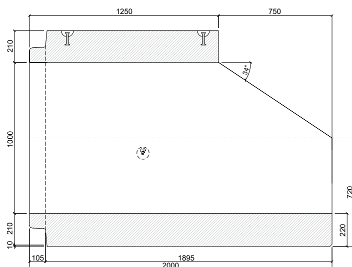
PATKOVÁ TROUBA TZP-ZP 100/200/125 SD
