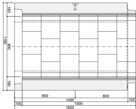
PATKOVÁ TROUBA TZP-SP 80/150 HDOC
