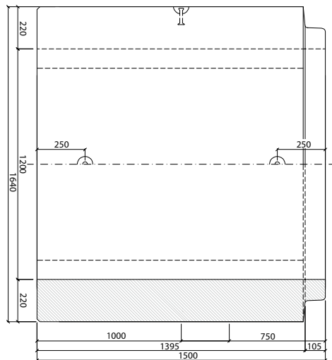
PATKOVÁ TROUBA TZP-ZP 120/150 KD
