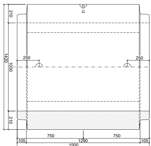
PATKOVÁ TROUBA TZP-SP 100/150 DD
