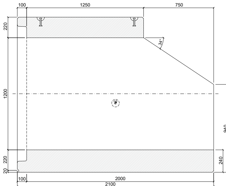
PATKOVÁ TROUBA TZP-ZP 120/200/125 SH
