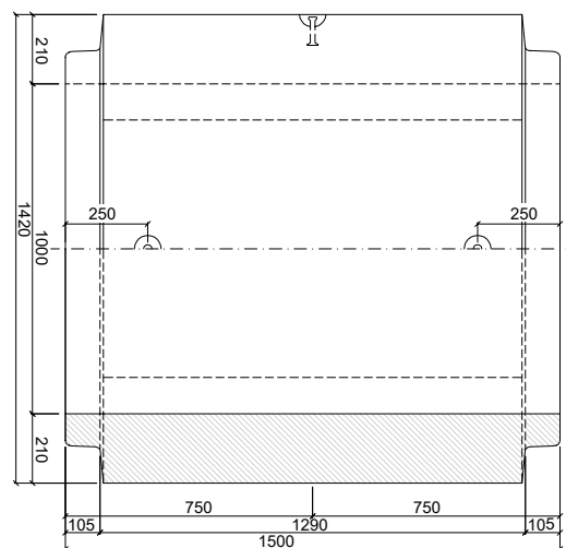
PATKOVÁ TROUBA TZP-ZP 100/150 DD
