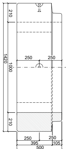
PATKOVÁ TROUBA TZP-ZP 100/50 KD
