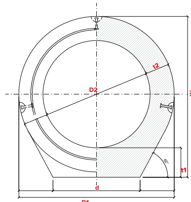
POHLED ČELNÍ / PŘÍČNÝ ŘEZ
