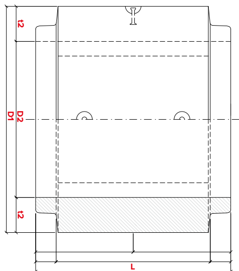
POHLED SESHORA / PODÉLNÝ ŘEZ
