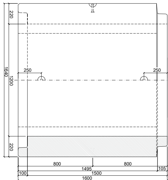
PATKOVÁ TROUBA TZP-SP 120/150 HD
