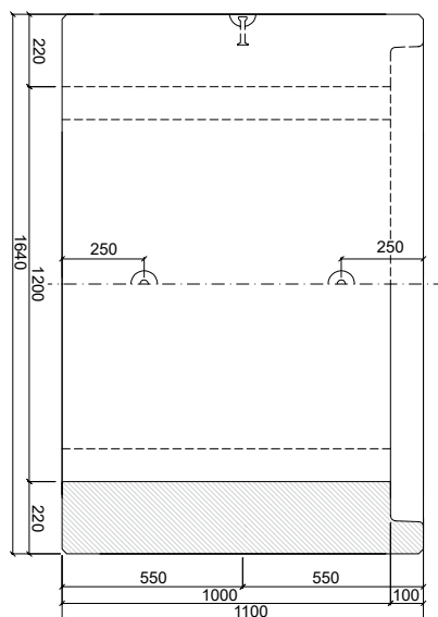
PATKOVÁ TROUBA TZP-ZP 120/100 KH
