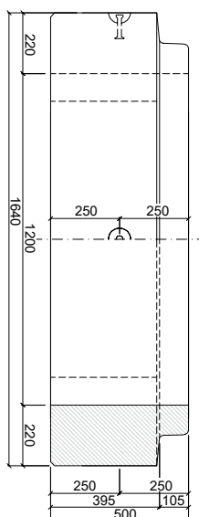
PATKOVÁ TROUBA TZP-ZP 120/50 KD
