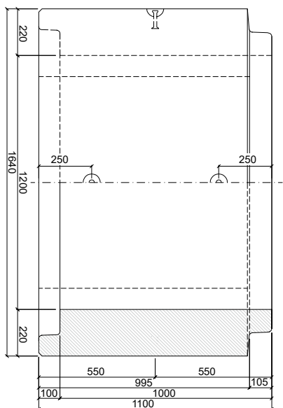
PATKOVÁ TROUBA TZP-ZP 120/200 HD
