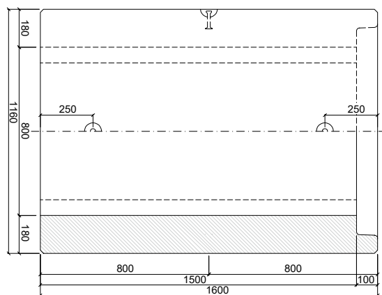
PATKOVÁ TROUBA TZP-SP 80/150 KH
