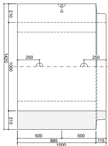
PATKOVÁ TROUBA TZP-ZP 100/100 KD
