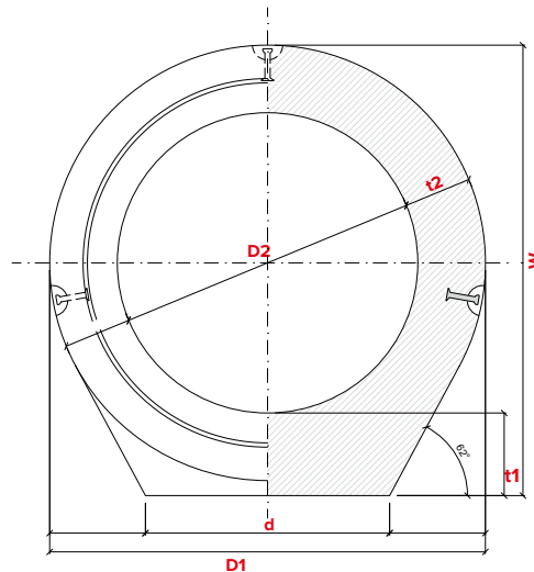
POHLED ČELNÍ / PŘÍČNÝ ŘEZ
