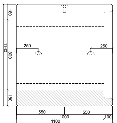
PATKOVÁ TROUBA TZP-ZP 80/100 KH
