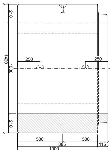
PATKOVÁ TROUBA TZP-SP 100/100 KD
