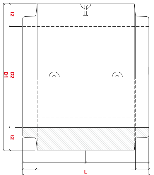
POHLED SESHORA / PODÉLNÝ ŘEZ
