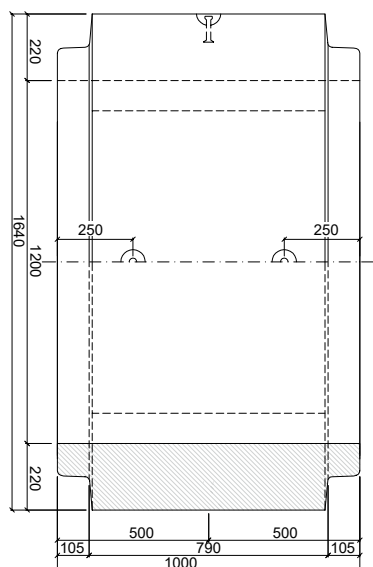
PATKOVÁ TROUBA TZP-ZP 120/100 DD
