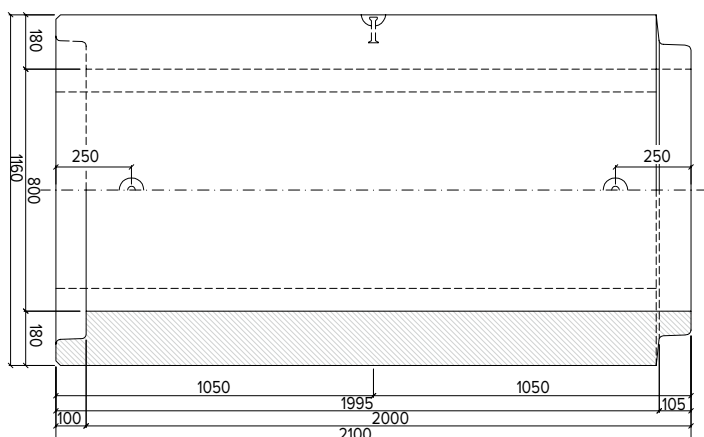
PATKOVÁ TROUBA TZP-ZP 80/200 HD
