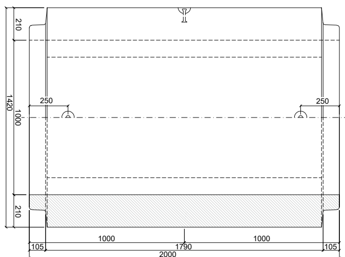
PATKOVÁ TROUBA TZP-SP 100/200 DD
