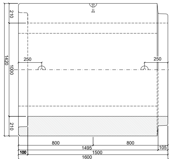
PATKOVÁ TROUBA TZP-ZP 100/150 HD
