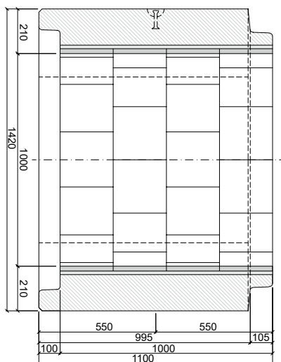
PATKOVÁ TROUBA TZP-SP 100/200 HDOC
