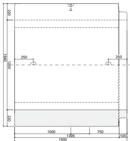
PATKOVÁ TROUBA TZP-SP 120/150 KD
