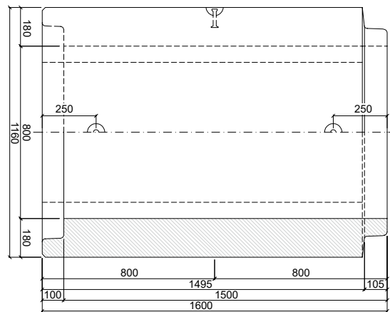
PATKOVÁ TROUBA TZP-SP 80/150 HD
