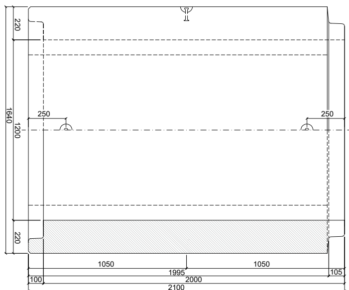
PATKOVÁ TROUBA TZP-SP 120/200 HD
