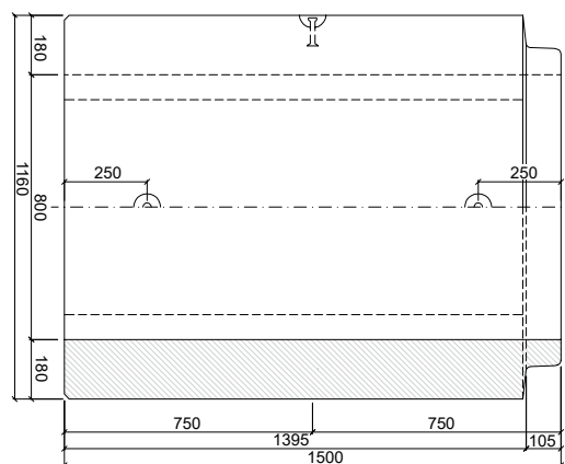
PATKOVÁ TROUBA TZP-SP 80/100 KD
