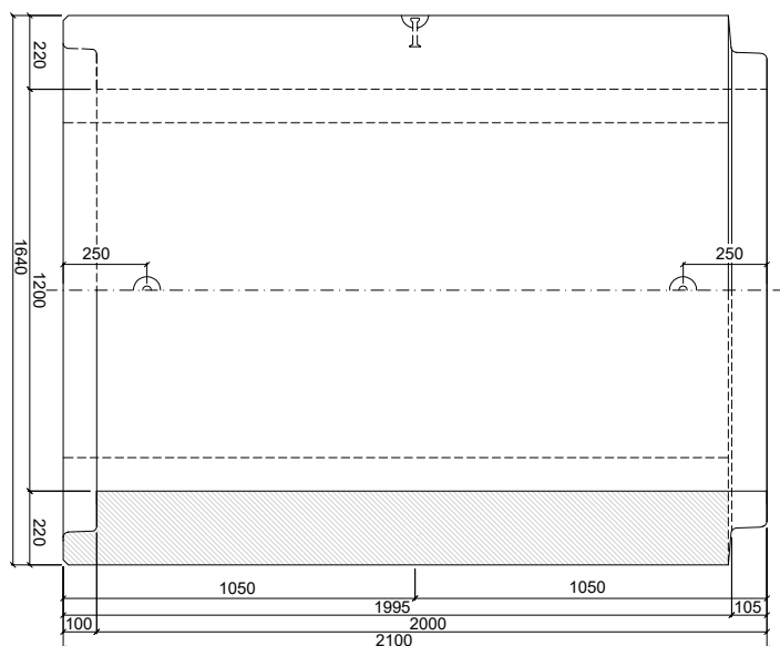
PATKOVÁ TROUBA TZP-ZP 120/200 HD
