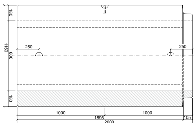
PATKOVÁ TROUBA TZP-SP 80/200 KD
