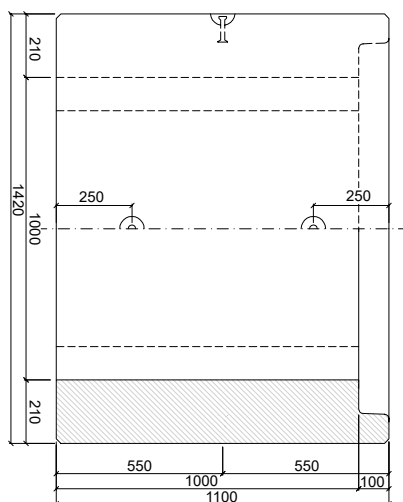
PATKOVÁ TROUBA TZP-ZP 100/100 KH
