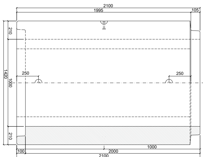
PATKOVÁ TROUBA TZP-SP 100/200 HD
