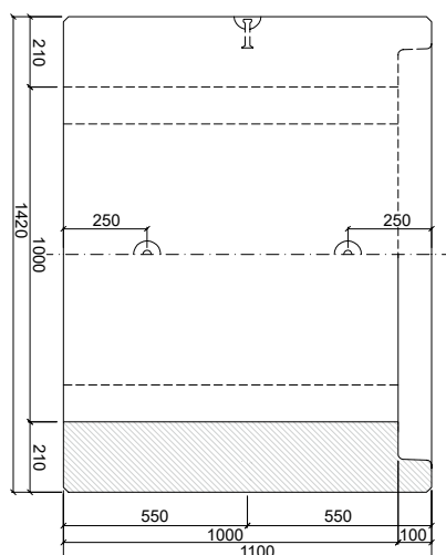
PATKOVÁ TROUBA TZP-SP 100/100 KH
