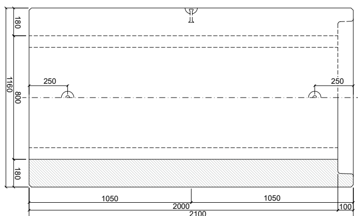
PATKOVÁ TROUBA TZP-SP 80/200 KH
