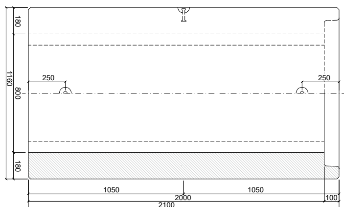
PATKOVÁ TROUBA TZP-ZP 80/200 KH
