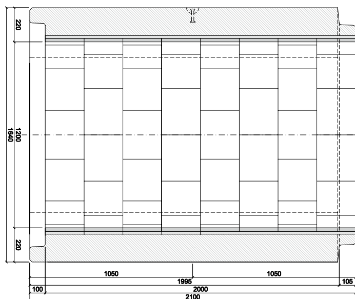
PATKOVÁ TROUBA TZP-SP 120/200 HDOC
