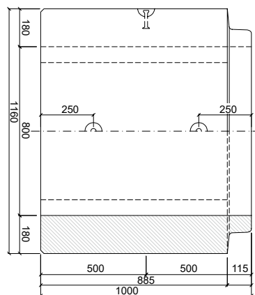
PATKOVÁ TROUBA TZP-ZP 80/100 KD
