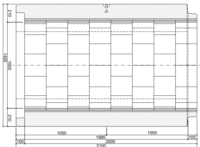
PATKOVÁ TROUBA TZP-SP 100/200 HDOC
