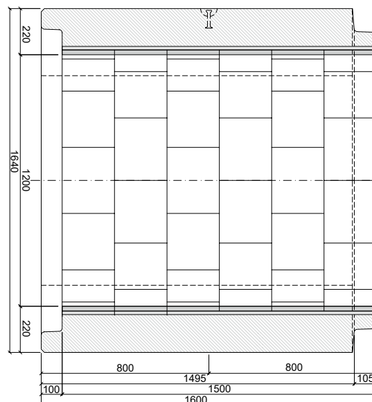
PATKOVÁ TROUBA TZP-SP 120/150 HDOC
