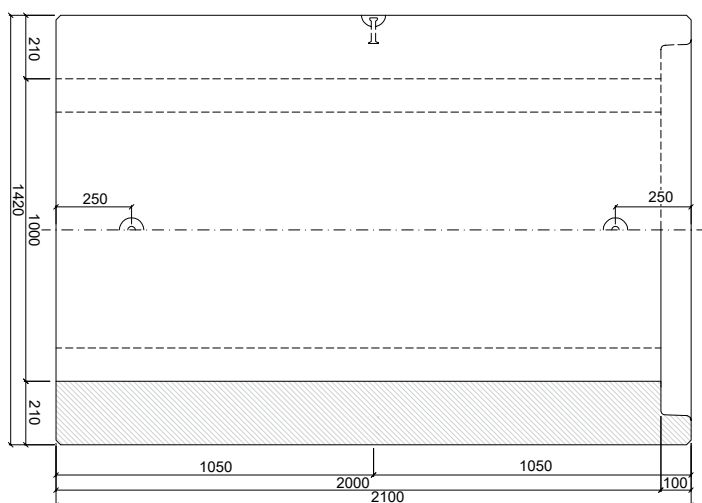
PATKOVÁ TROUBA TZP-SP 100/200 KH
