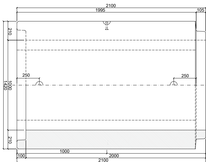
PATKOVÁ TROUBA TZP-ZP 100/200 HD
