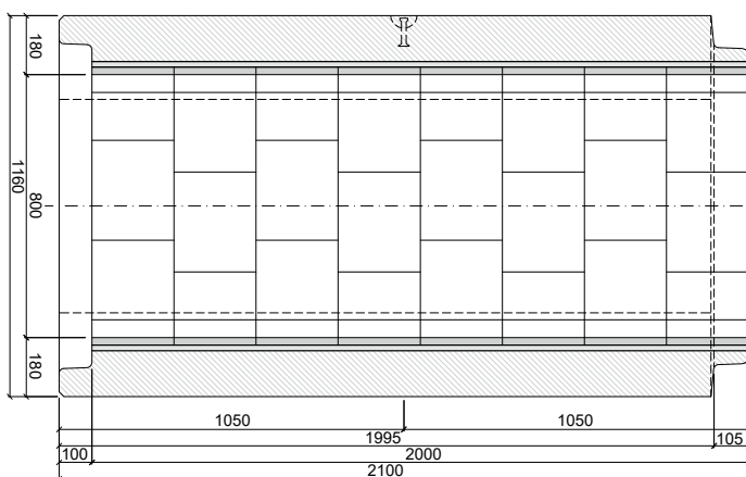
PATKOVÁ TROUBA TZP-SP 80/200 HDOC
