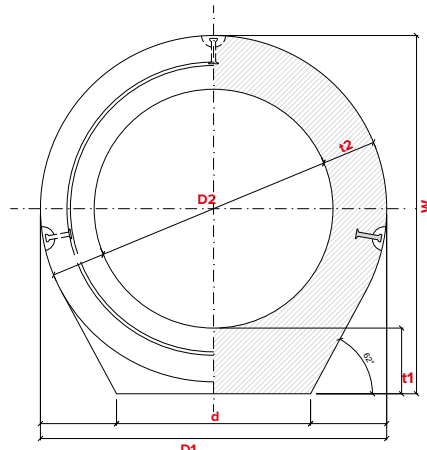
POHLED ČELNÍ / PŘÍČNÝ ŘEZ
