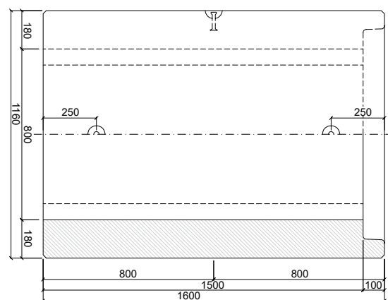
PATKOVÁ TROUBA TZP-ZP 80/150 KH
