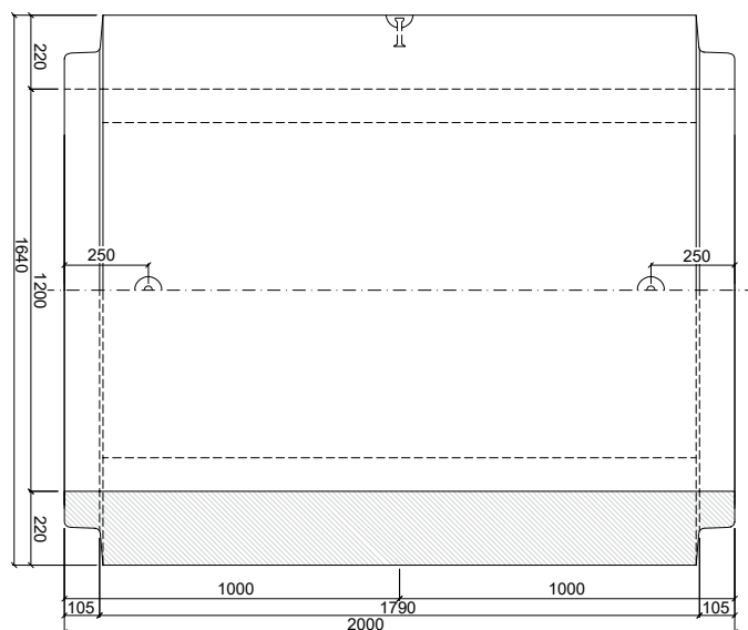
PATKOVÁ TROUBA TZP-SP 120/200 DD
