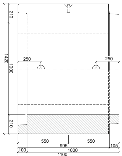
PATKOVÁ TROUBA TZP-ZP 100/100 HD
