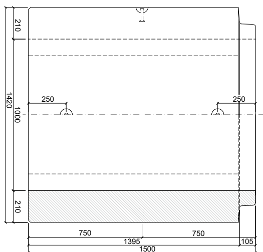
PATKOVÁ TROUBA TZP-ZP 100/150 KD
