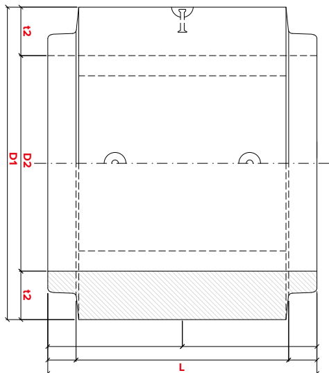
POHLED BOČNÍ / PODÉLNÝ ŘEZ
