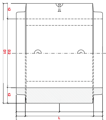
POHLED SESHORA / PODÉLNÝ ŘEZ
