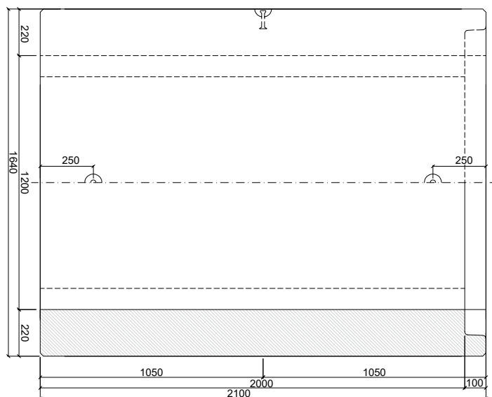
PATKOVÁ TROUBA TZP-SP 120/200 KH
