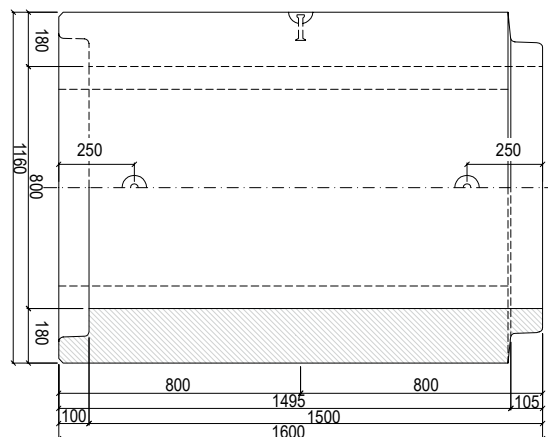
PATKOVÁ TROUBA TZP-ZP 80/150 HD
