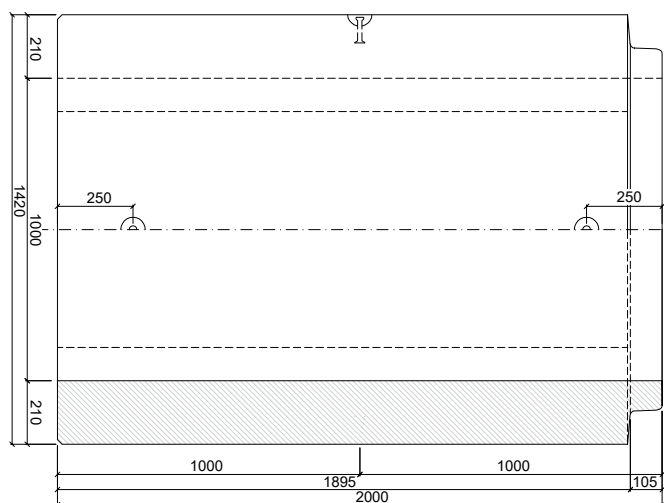
PATKOVÁ TROUBA TZP-SP 100/200 KD
