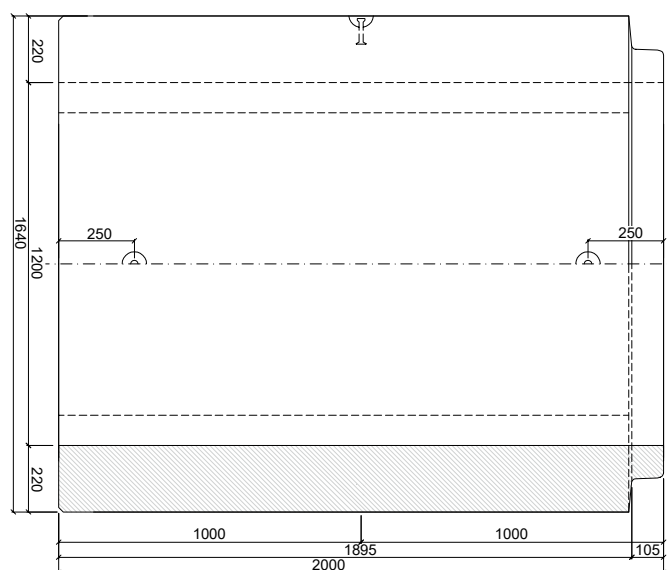
PATKOVÁ TROUBA TZP-SP 120/200 KD
