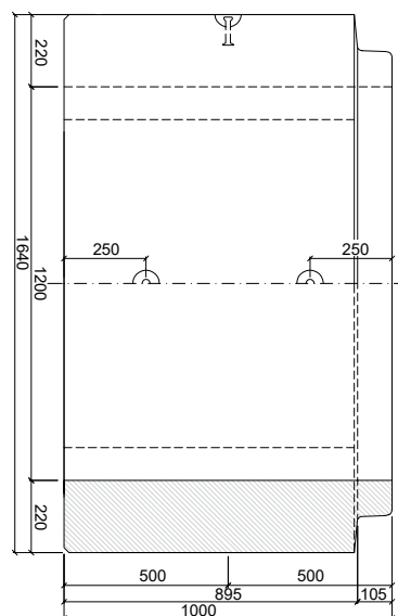
PATKOVÁ TROUBA TZP-SP 120/100 KD
