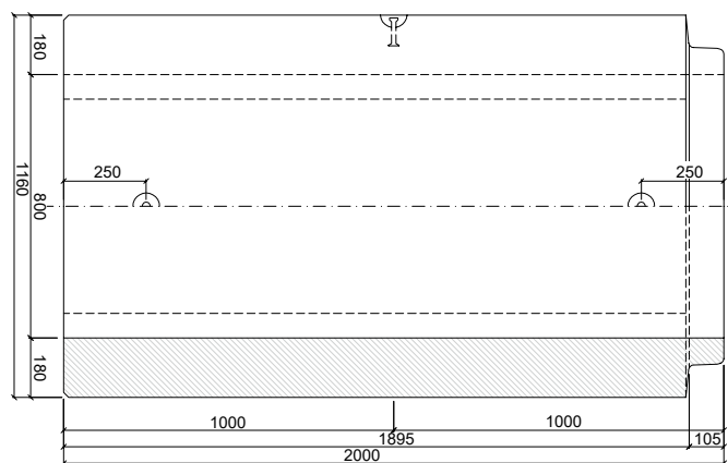
PATKOVÁ TROUBA TZP-ZP 800/200 KD
