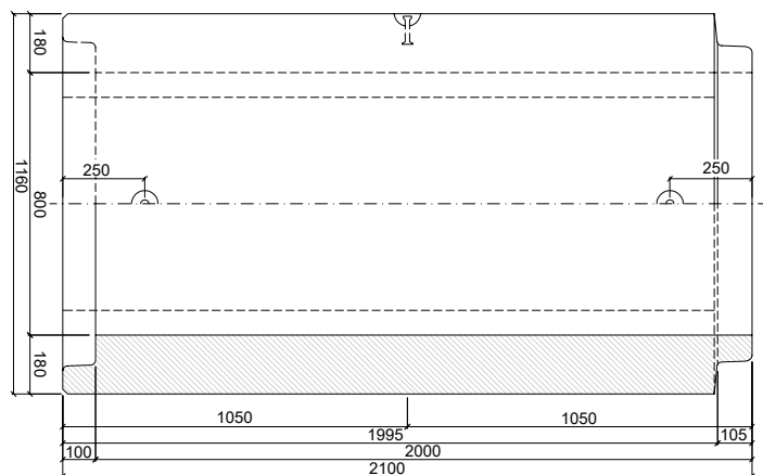
PATKOVÁ TROUBA TZP-SP 80/200 HD
