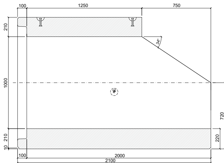
PATKOVÁ TROUBA TZP-ZP 100/200/125 SH
