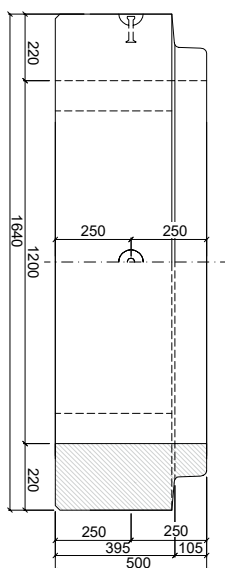
PATKOVÁ TROUBA TZP-SP 120/50 KD
