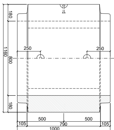
PATKOVÁ TROUBA TYP-ZP 80/100 DD
