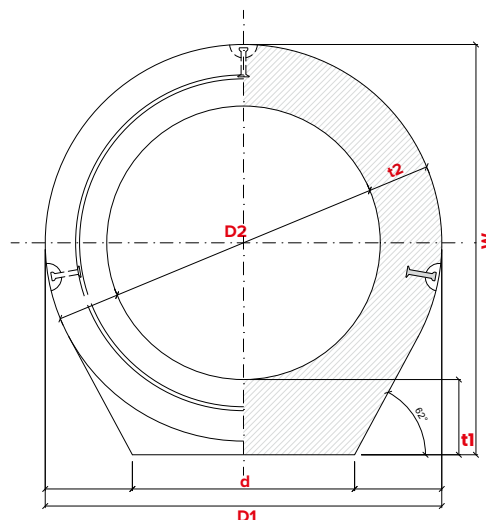
PŘÍČNÝ ŘEZ
