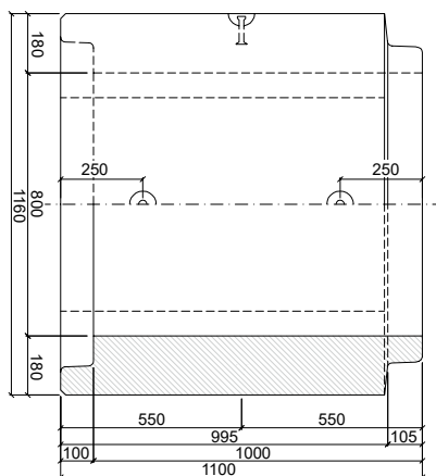
PATKOVÁ TROUBA TZP-SP 80/100 HD
