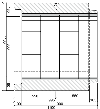
PATKOVÁ TROUBA TZP-SP 80/100 HDOC
