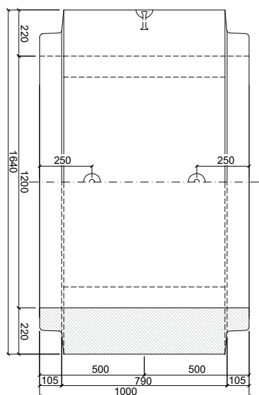
PATKOVÁ TROUBA TZP-SP 120/100 DD
