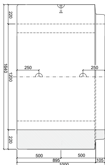
PATKOVÁ TROUBA TZP-ZP 120/100 KD
