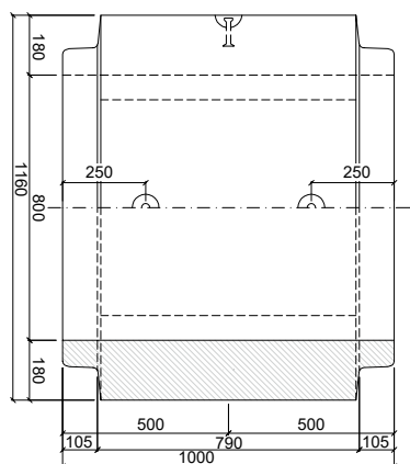
PATKOVÁ TROUBA TZP-SP 80/200 DD
