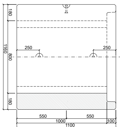
PATKOVÁ TROUBA TZP-SP 80/100 KH
