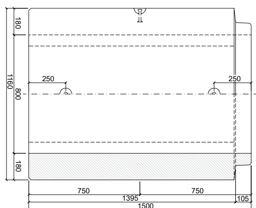
PATKOVÁ TROUBA TZP-SP 80/150 KD
