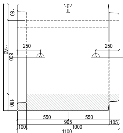
PATKOVÁ TROUBA TZP-ZP 80/100 HD
