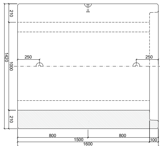
PATKOVÁ TROUBA TZP-ZP 100/150 KH
