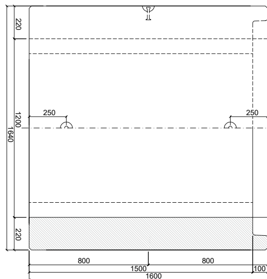
PATKOVÁ TROUBA TZP-ZP 120/150 KH
