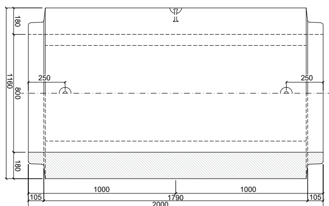
PATKOVÁ TROUBA TZP-SP 80/200 DD
