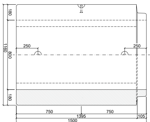
PATKOVÁ TROUBA TZP-ZP 800/150 KD
