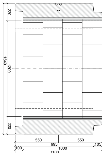
PATKOVÁ TROUBA TZP-SP 120/100 HDOC
