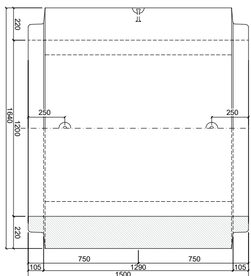
PATKOVÁ TROUBA TZP-SP 120/150 DD
