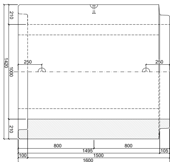
PATKOVÁ TROUBA TZP-SP 100/150 HD
