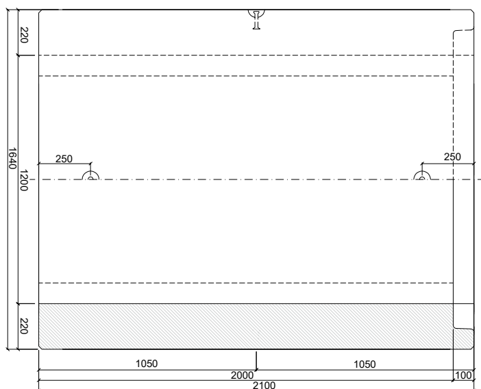
PATKOVÁ TROUBA TZP-ZP 120/200 KH
