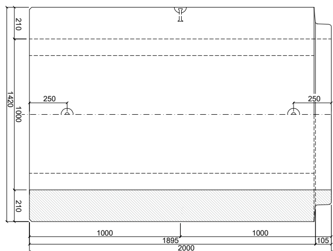
PATKOVÁ TROUBA TZP-ZP 100/200 KD
