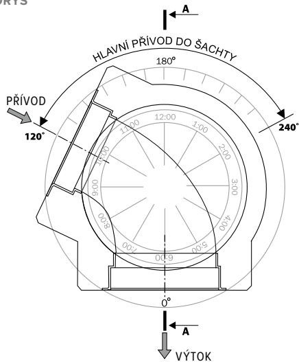
PŮDORYS
