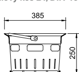
kalový koš B1, DIN 4052
