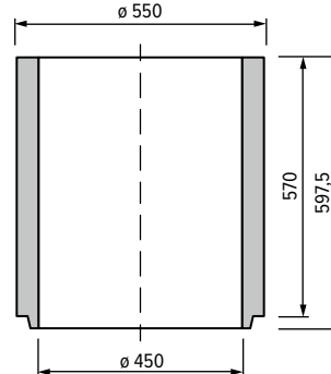
TBV-Q 5d/450/570 skruž horní
