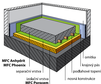
Topný potěr
