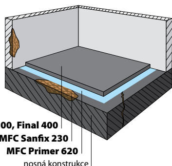
Sanace lokálních výtluků a prasklin
