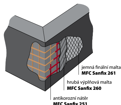
Systém sanace železobetonových konstrukcí
