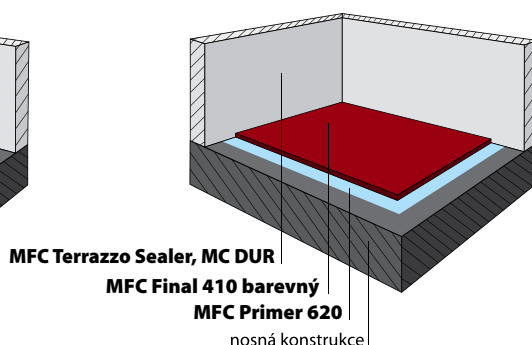
Povrchová úprava podlahy MFC Final 410
