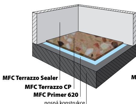
Povrchová úprava podlahy MFC Micro Terrazzo CP
