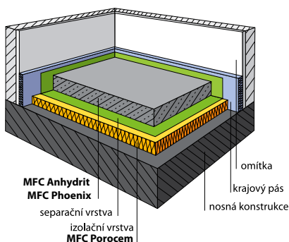
Potěr na izolační vrstvě
