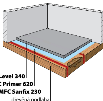
Vyrovnávání podkladu při rekonstrukci dřevěné podlahy
