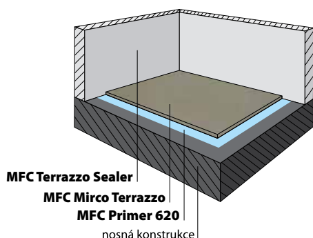
Povrchová úprava podlahy MFC Micro Terrazzo
