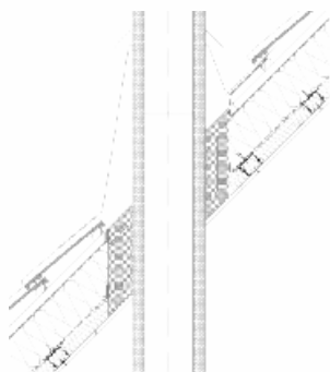
Parotěsný prostop v šikmé střeše (GPK10)
