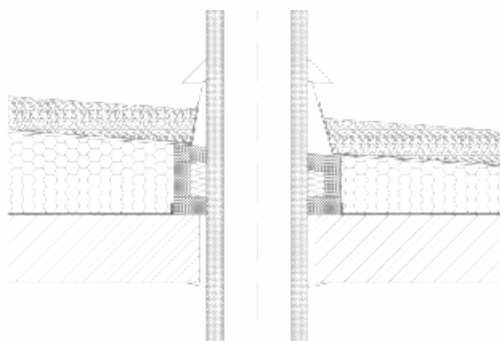
Parotěsný prostop v zelené střeše (GPKL)
