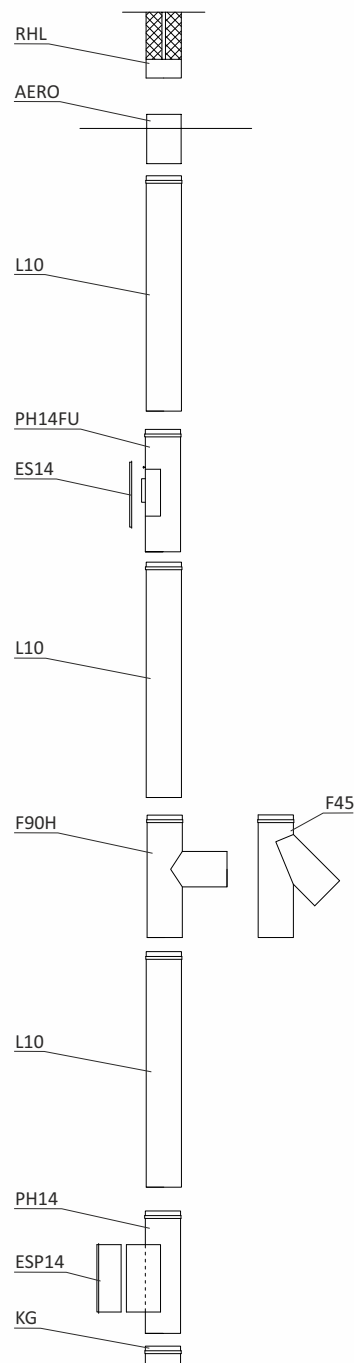
Vložkování nerez pevný podtlak
