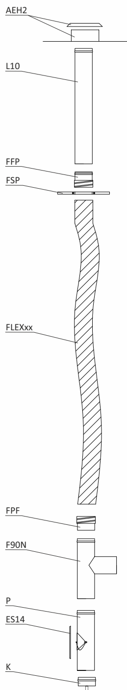
Vložkování nerez flexi přetlak
