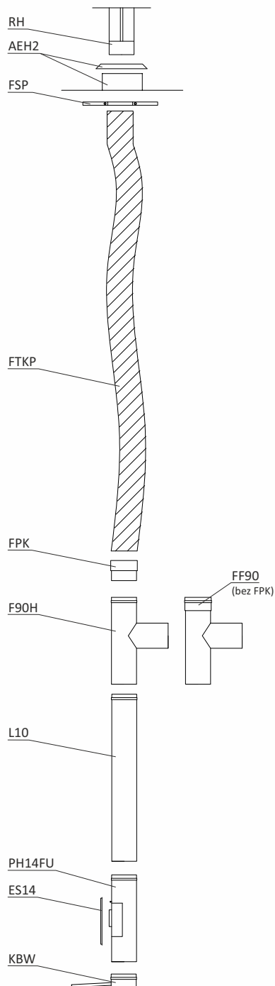
Vložkování nerez flexi podtlak
