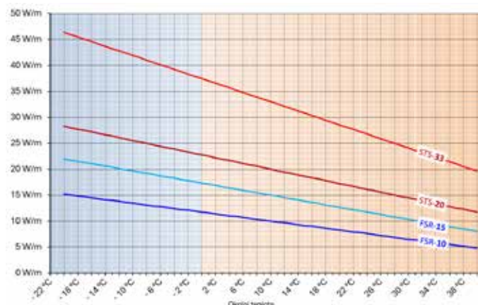
Graf teplota / výkon
