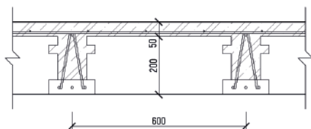
ŘEZ STROPNÍ KONSTRUKCE
