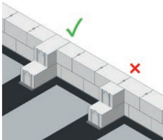
Obrázek správného napojení na vazbu
