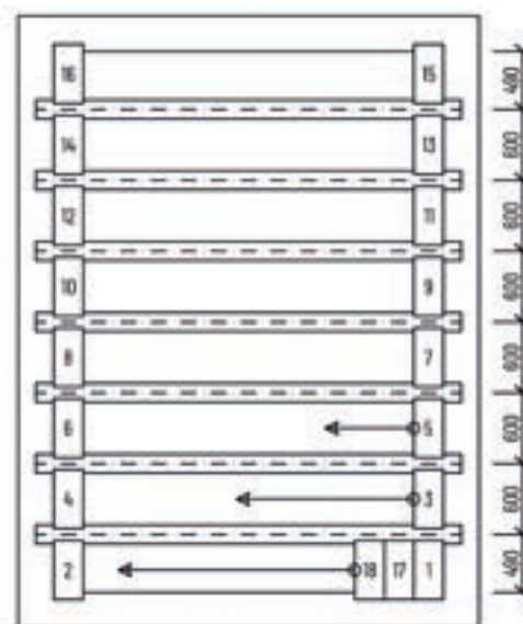
KLADENÍ NOSNÍKŮ A VLOŽEK
