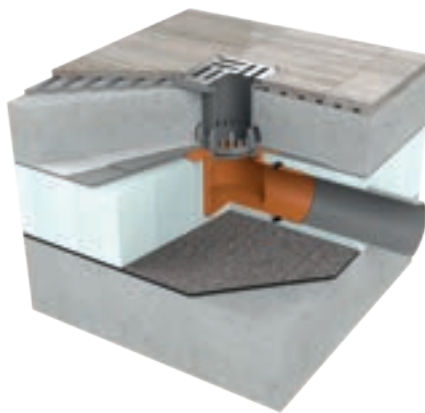
Skladba balkonu s drenážní vrstvou
