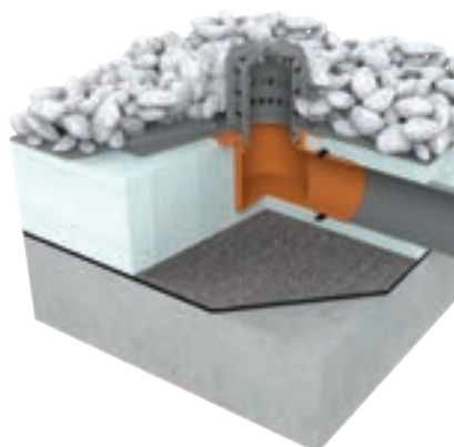
Skladba balkonu s vrstvou kačírku
