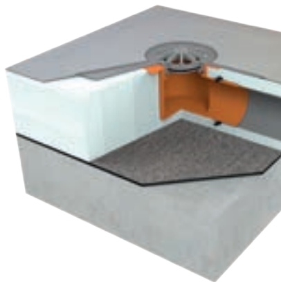
Skladba balkonu s pochozí střešní folií
